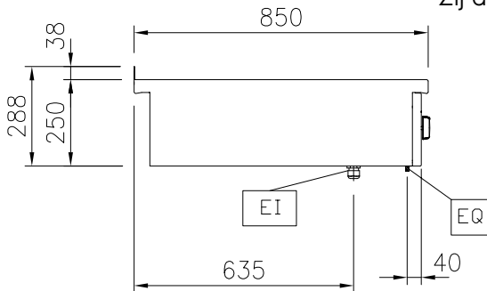
Zij aanzicht
