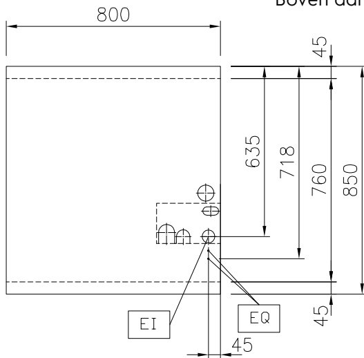
Boven aanzicht
